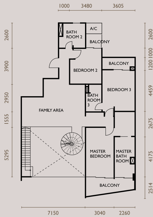
TYPE D4 - UPPER
